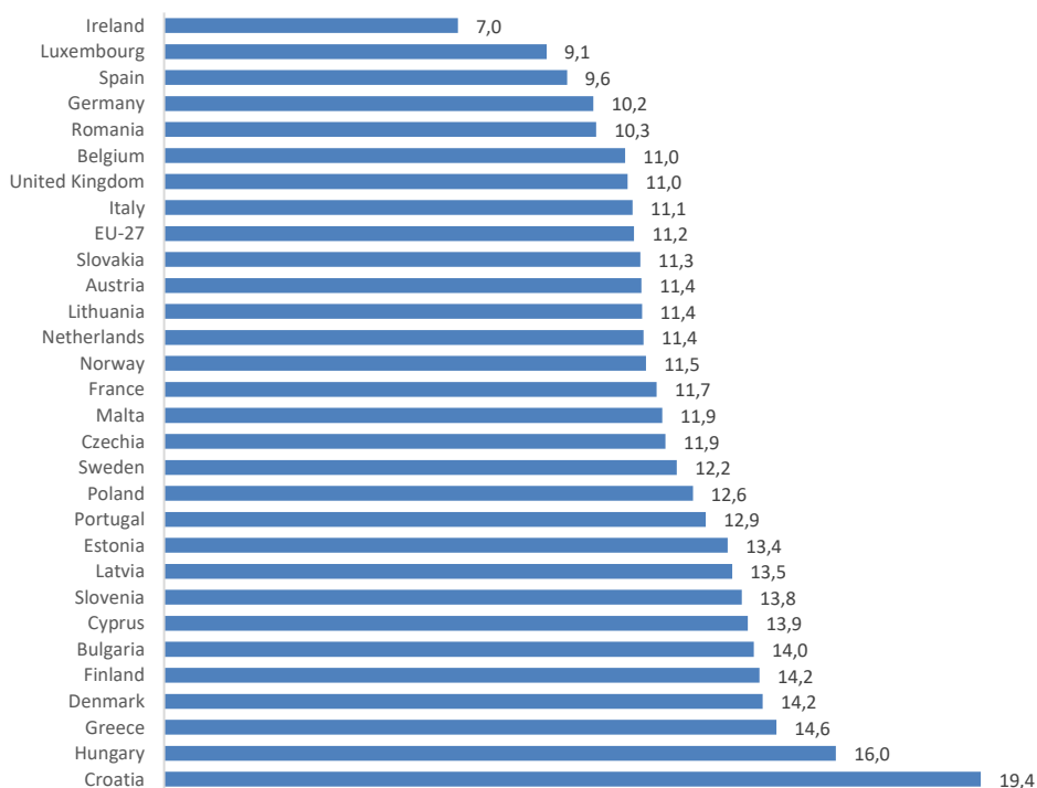
Figura 14 - La Pressione Fiscale sul consumo in Italia. Anno 2018. (Valori %)
