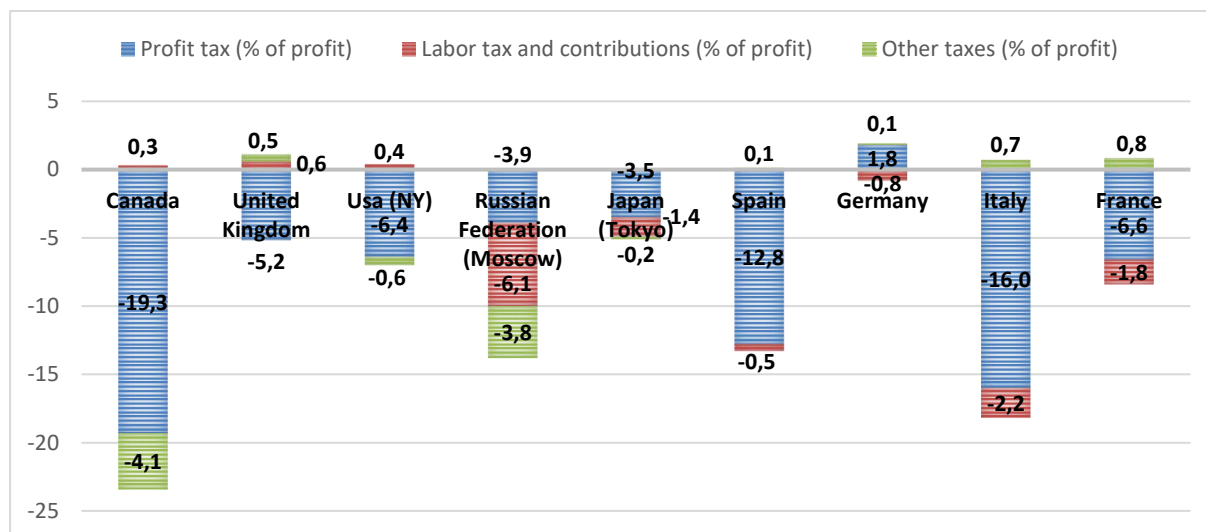
Figura 20 - Variazioni tra il 2006 e il 2020 delle singole componenti del TTCR dei paesi del G8 più Russia. (Valori %)
