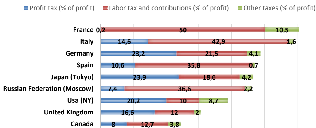
Figura 19 - Le principali componenti del TTCR nel G8. DB2020. (Valori %)
